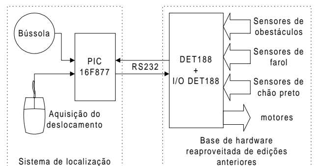
Fig. 5 – Esquema geral do hardware
