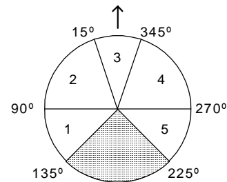
Fig. 9 – Divisão do campo de detecção de farol
